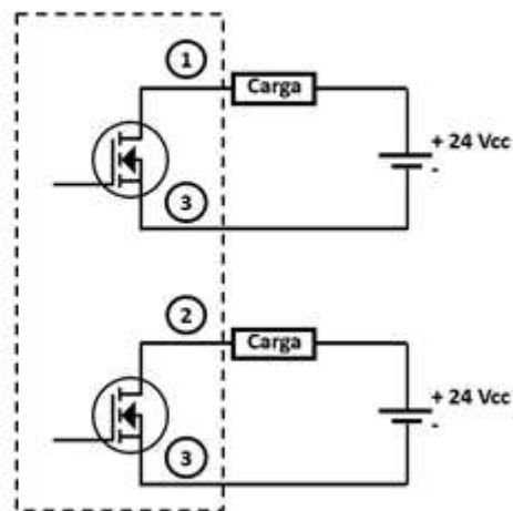
SAÍDAS DIGITAIS PARA ALARMES /SEGURANÇA
